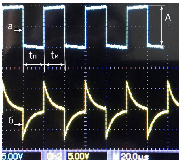
Рисунок 2. Осциллограммы импульсных сигналов: а — сигнал прямоугольной формы, б — сигнал, измененный дифференцирующей цепью Figure 2. Oscillograms of pulse signals: a — rectangular signal, b — signal modified by the differentiating circuit
